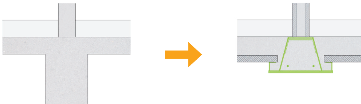
PREFABRIKOVANÝ STROP SO STENAMI Z CLT PANELOV
